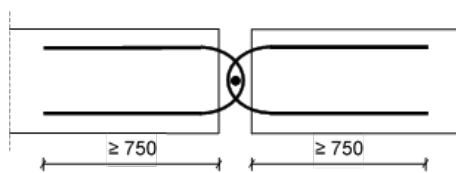
Bild: Vertikale Stoßfuge in Wandebene bei Brandwänden
